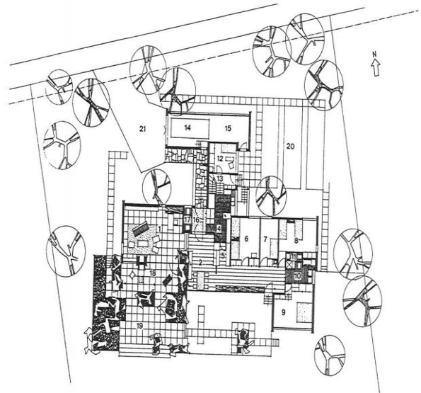
2 Grundriss
